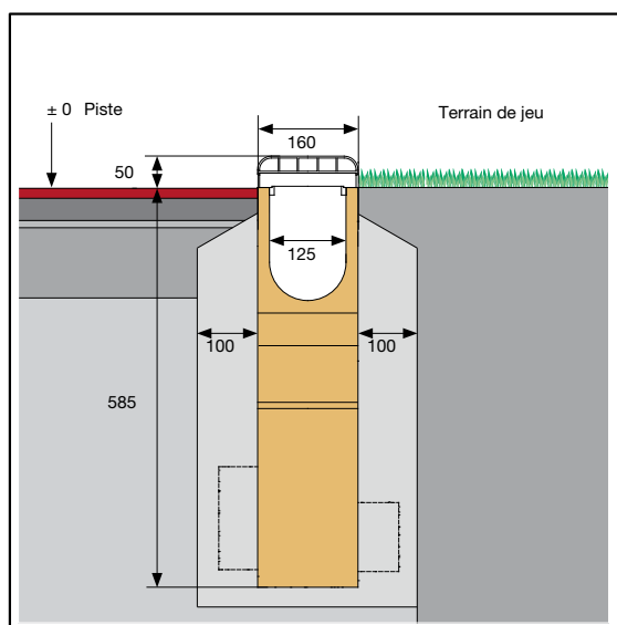
ANRIN SPORT système de drainage 125 Avaloir 125 J, sans rebord d'un côté
