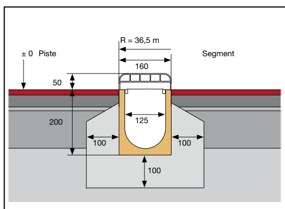
ANRIN SPORT système de drainage 125 caniveau 125 A/B
