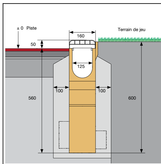
ANRIN SPORT système de drainage 125 Avaloir 125 K, avec 4 cm rebord d'un côté
