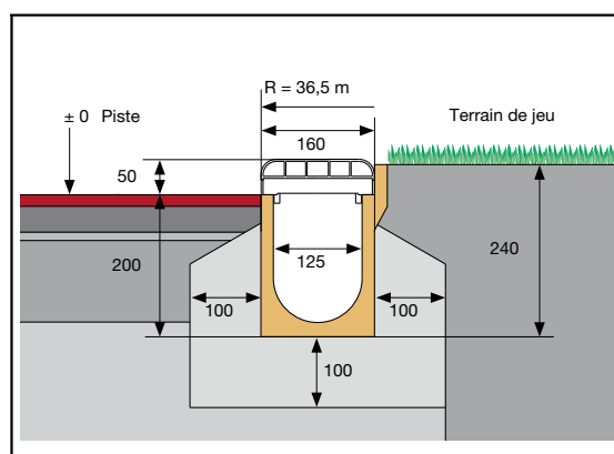
ANRIN SPORT système de drainage 125 caniveau 125 E/F
