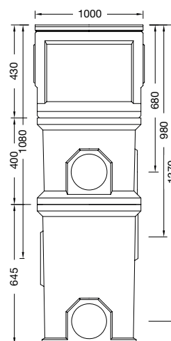
SF-200 sandfång med slitsat segjärnsgaller bk. F900 1
