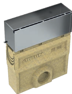
Access topp Z-100 S kombinerad med ränna Z-100 Nr. 055
