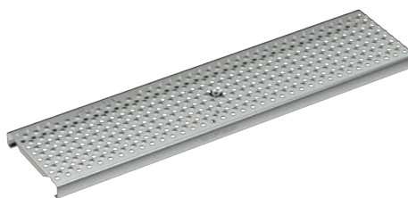
Perforerat galler, galvaniserad, rostfritt stål Belastningsklass: A15, C250 , Längd: 50 cm, 100 cm, Ø 6 mm
