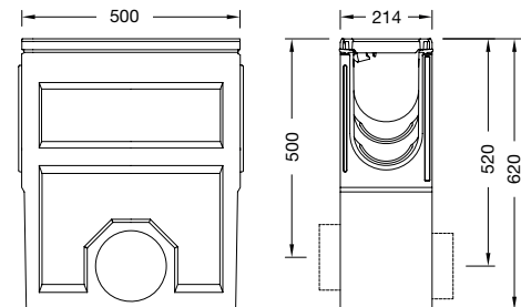
SF-150 sandfång med slitsat segjärnsgaller bk. F900 1
